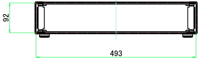
A-A ( 1 : 7 )
